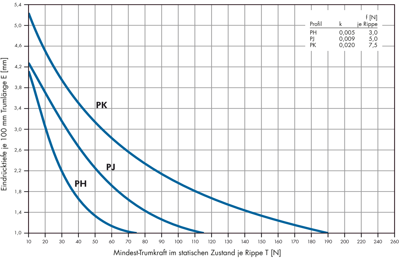
Diagramm 2: Vorspannungskennlinien
