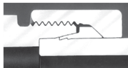
Profilring – Keine Deformation bei Überanzug
